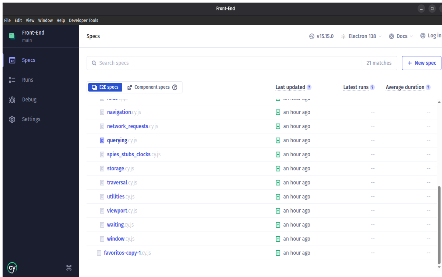
Figura A.9 – Lista de especificações E2E no Cypress Test Runner
